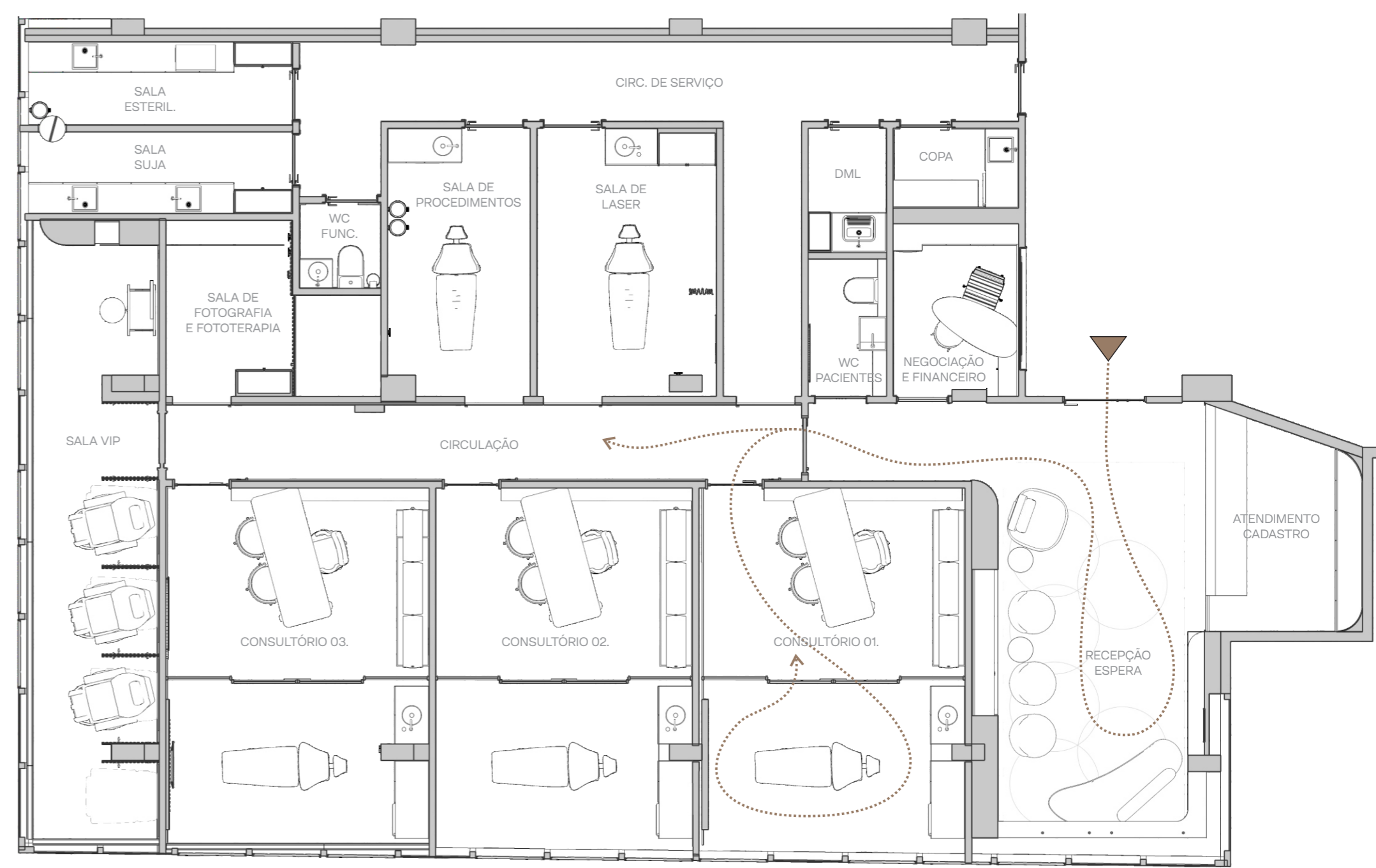
PLANTA BAIXA - LAYOUT CONSULTÓRIO
