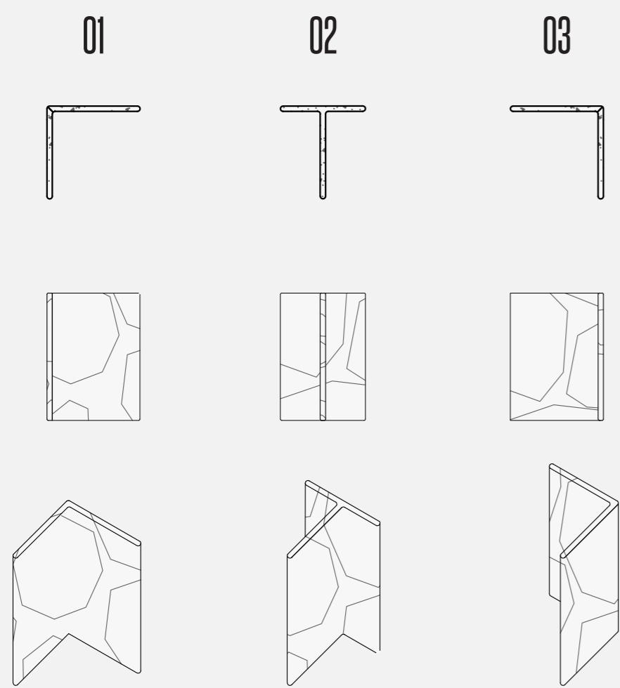
MÓDULOS ESC:1/20
