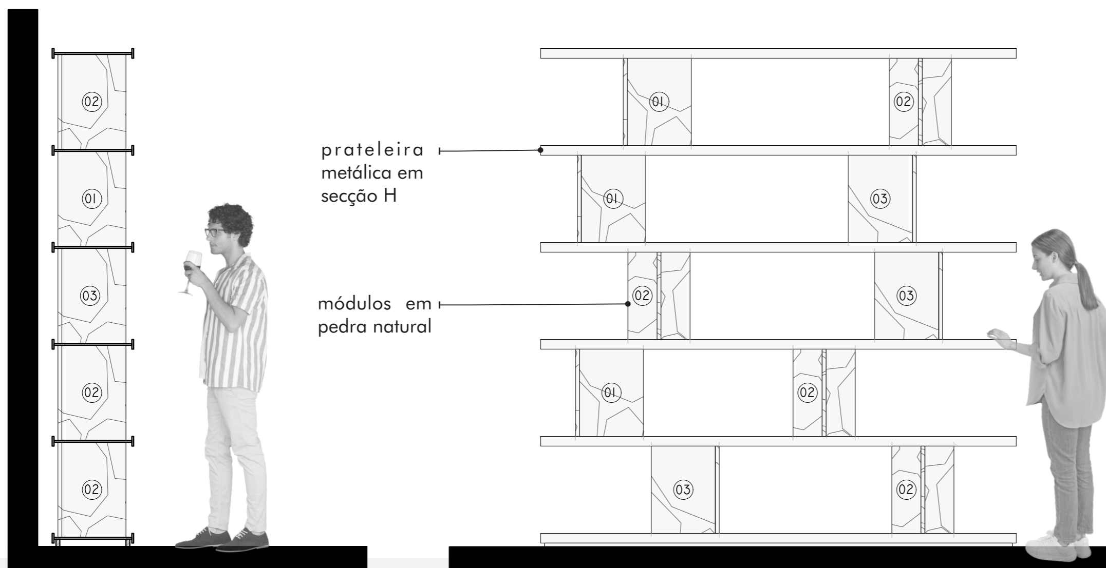
VISTA LATERAL ESC:1/20
