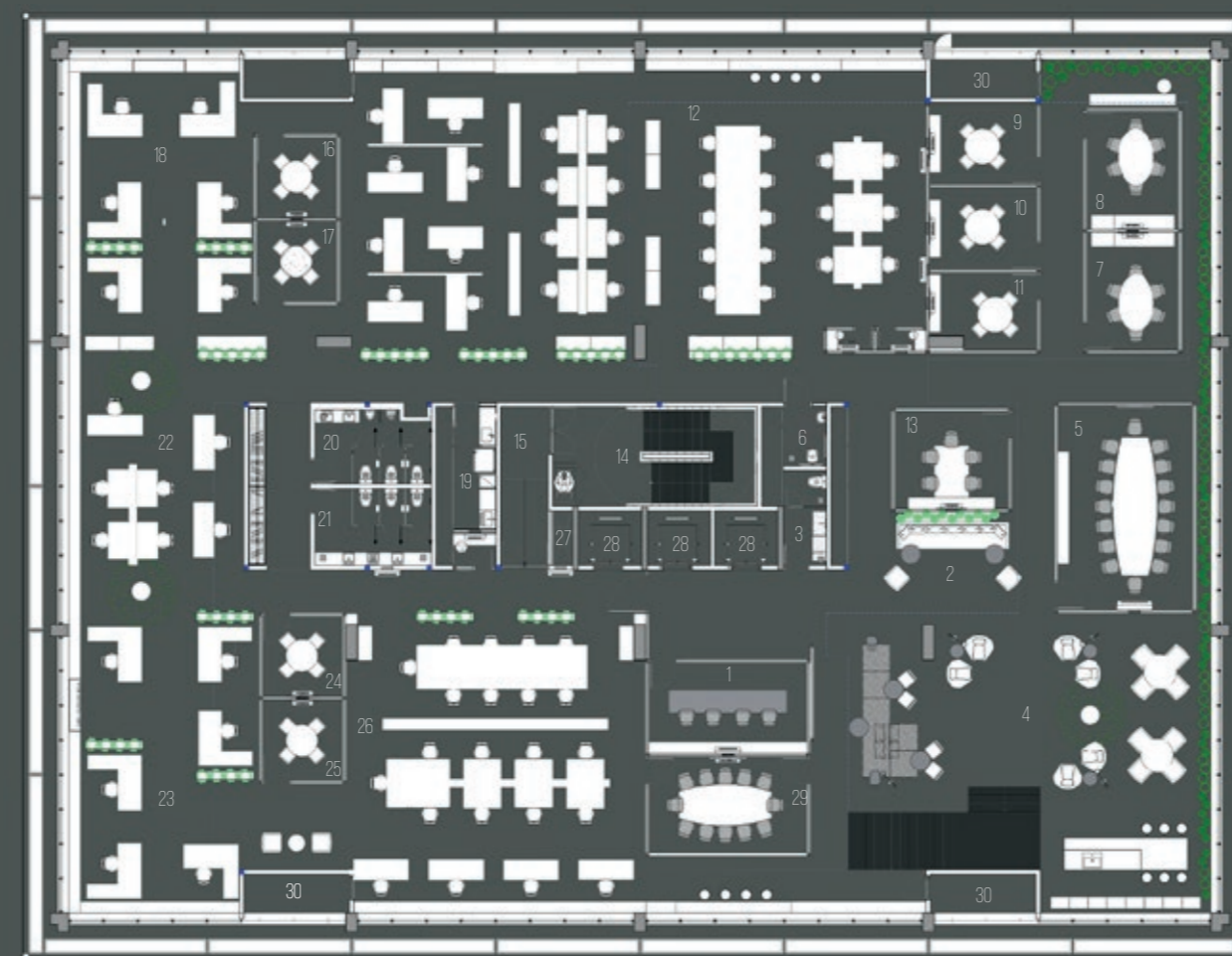
PRIMEIRO PAVIMENTO
